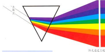
阳光通过三棱镜
